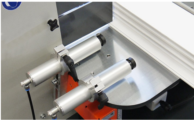
Fraiseuse en bout AF 222/02
